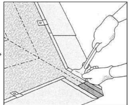
3. 縦はげに水返し用のアダ折をする。
