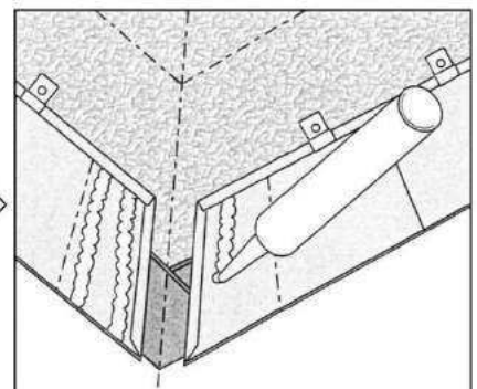
6. はやぶき本体と廻し葺一段目の重ね部分にコーキングをする。
