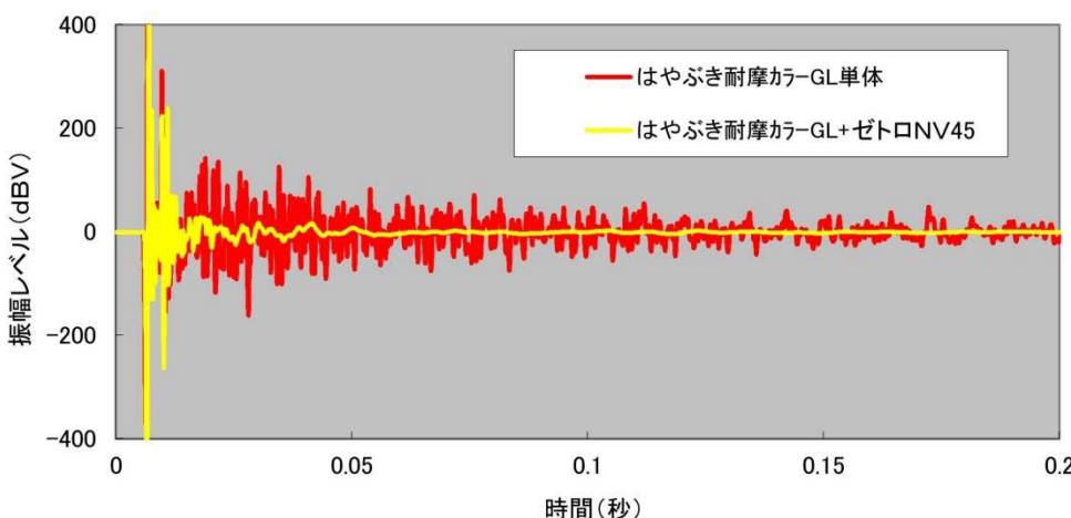
はやぶき耐摩カラー-GLに対するゼトロNV45貼付による振動減衰特性
