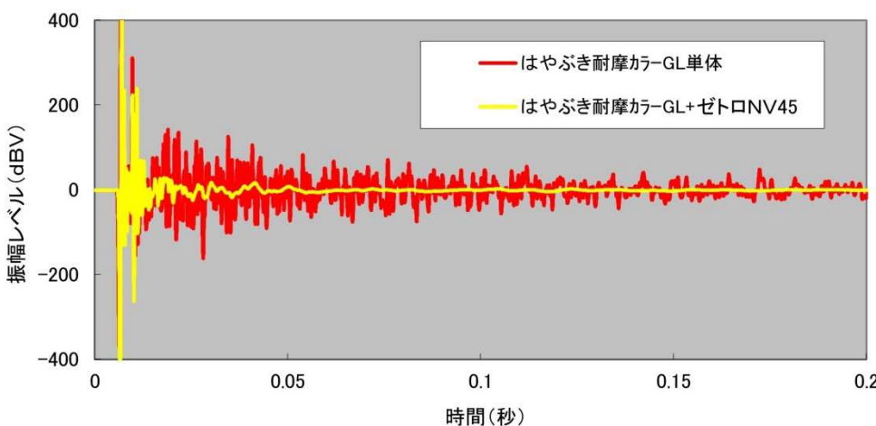
はやぶき耐摩カラー-GLに対するゼトロNV45貼付による振動減衰特性
